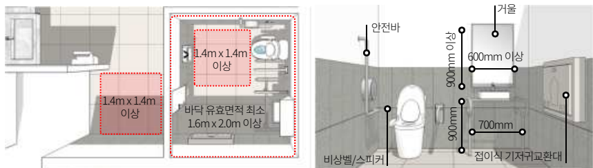
장애인화장실(다목적화장실) 공간설계 기준
