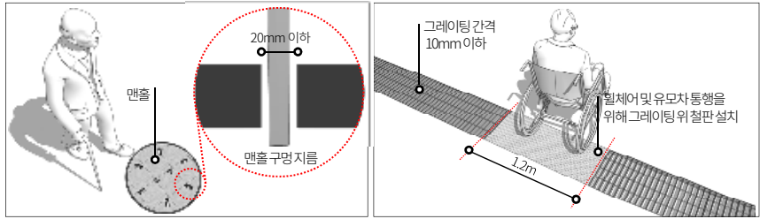
맨홀의 구멍 지름 기준 그레이팅 연속 설치 구간에는 폭 1.2m의 철판 설치
