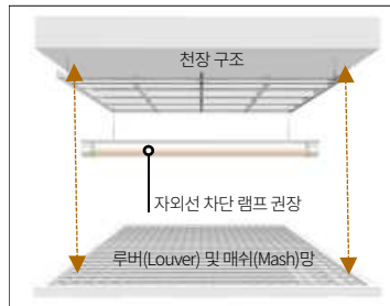
루버(Louver) 및 매쉬(Mash)망 구조도
