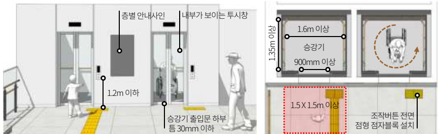
승강기 전면 공간예시 승강기 내·외부 유효공간 설계기준
